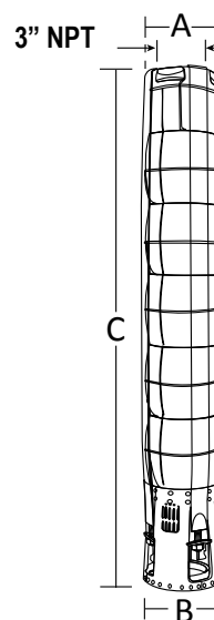
Acoplamiento NEMA 6"
