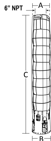
Acoplamiento NEMA 10" Fig. 2
