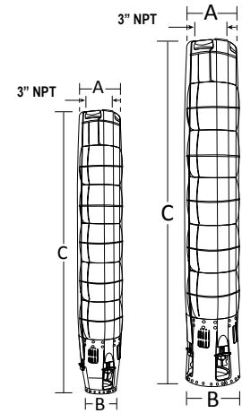
Acoplamiento NEMA 4" Fig. 1 Acoplamiento NEMA 6" Fig. 2
